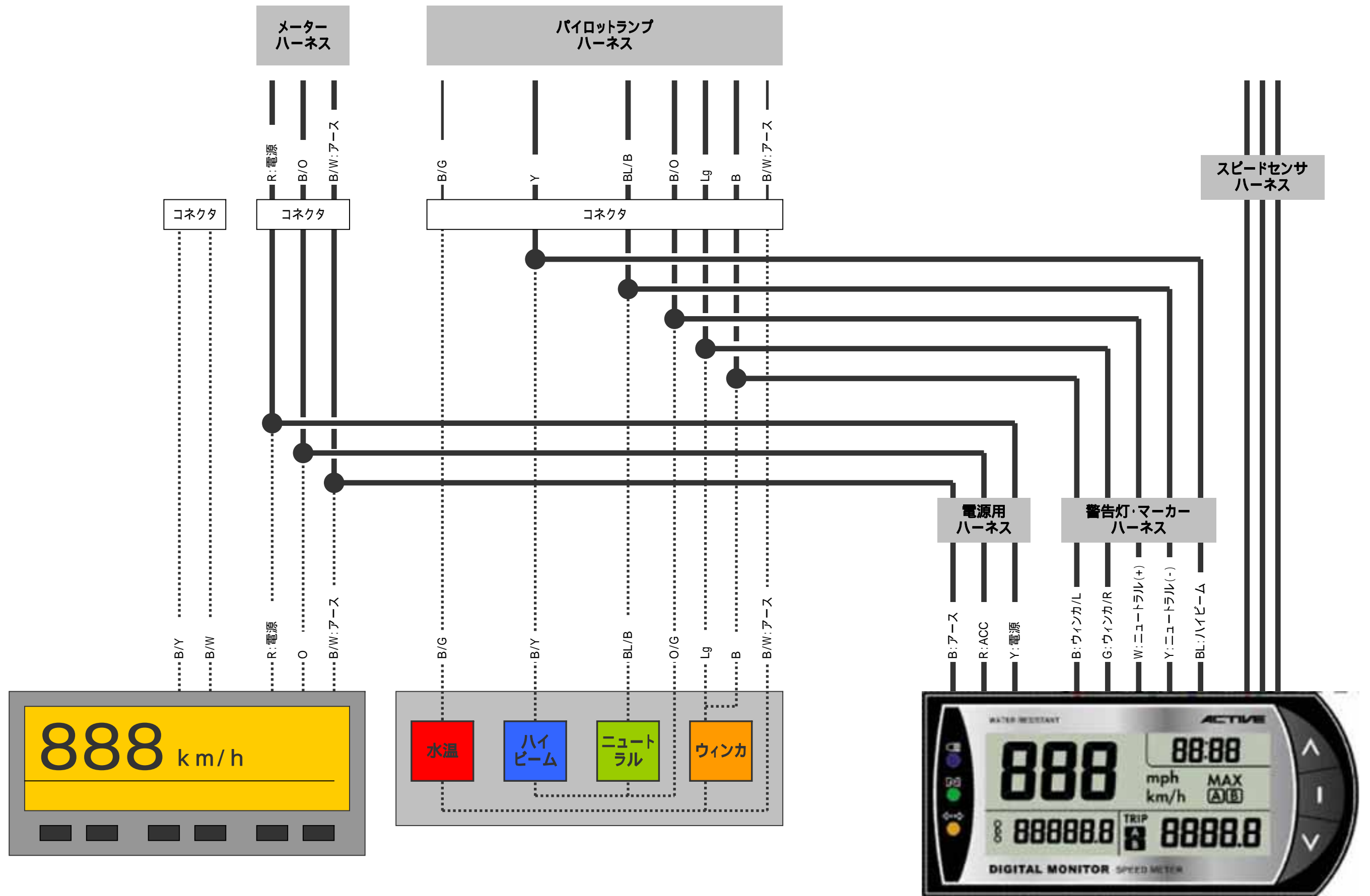
DR-Z400SMノーマルメーター側配線
